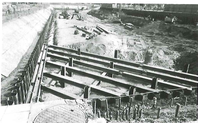
Hình ảnh thi công hố đào mở
