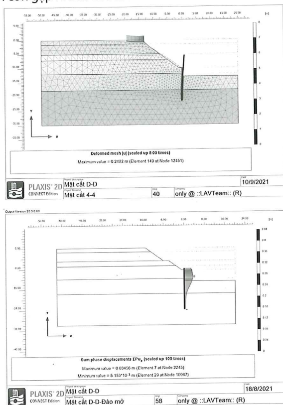
Hình ảnh tính toán hố đào mở bằng phần mềm Palxis
