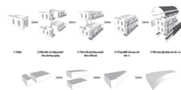
Hình 11. Phương án công trình phát triển theo mô đun
