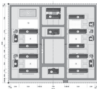
Hình 6. Tổng mặt bằng một doanh trại điển hình
