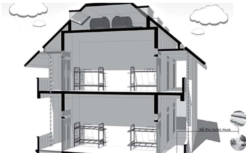
Hình 12. Phương án công trình điển hình
